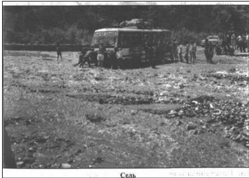
Сель
