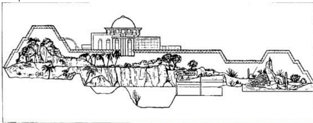
Рис. 1.8. Поперечный срез искусственной биосферы II (по: Allen, Nelson, 1986).
