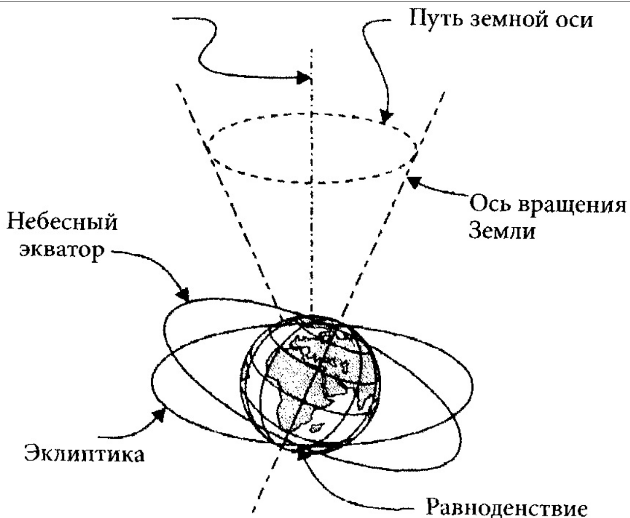
Рис. 2. Схема прецессии
