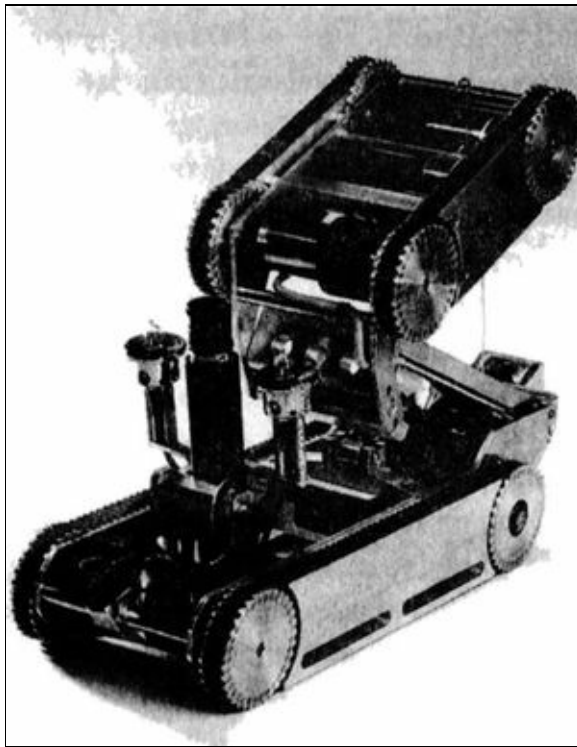
Робот UPUAUT, сконструированный Рудольфом Гантенбринком
